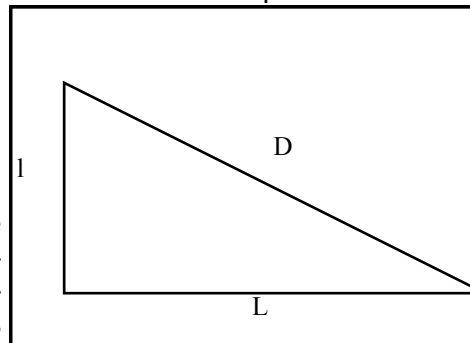
Figure 4 : utilisation du théorème de Pythagore : (l \times l) + (L \times L) = (D \times D) . Il faut donc mesurer par exemple 3 m sur une ligne, 4 sur l'autre, la distance entre les points doit être de 5 m si les lignes sont perpendiculaires. Doubler les longueurs pour plus de précision (6, 8 et 10 m)
